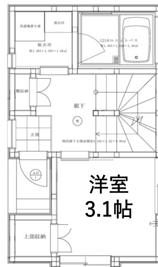
一階
